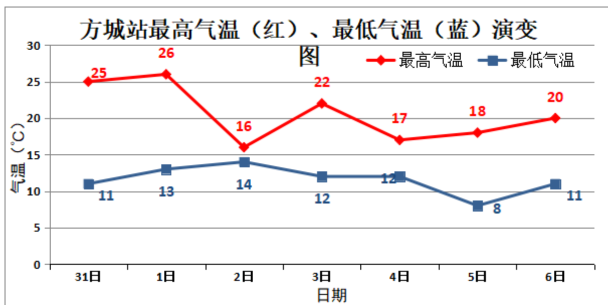
图1 2024年3月31日~4月6日方城站最高气温（红线）、最低气温（蓝线）预报图（℃）
